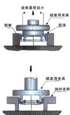
骨架油封不正确的组装
