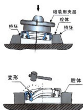
骨架油封不正确的组装
