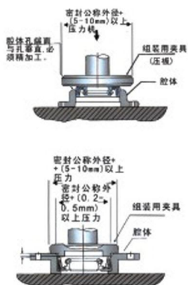
骨架油封的正确组装
