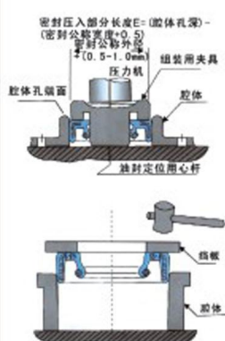
骨架油封的正确组装
